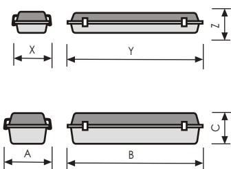
Dimensões (mm)
